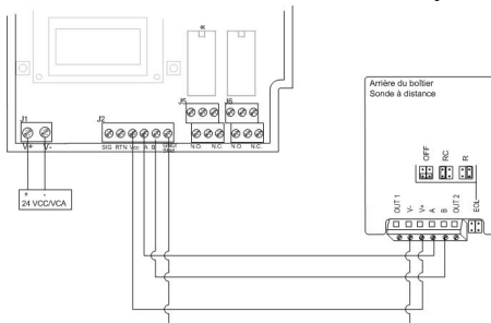
Illustration 2. Connexion de l'unité principale au détecteur à distance
